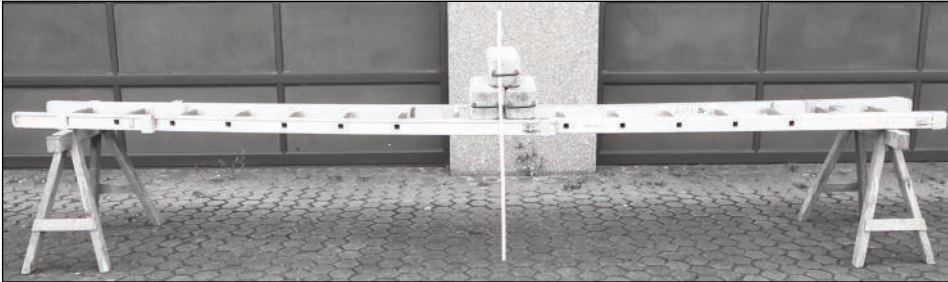
Prüfung einer 2-teiligen Steckleiter mit einem Prüfungsgewicht von 30 kg auf Durchbiegung. Zwei solcher zusammengesteckten Leiterteile ergeben eine 4-teilige Steckleiter.
